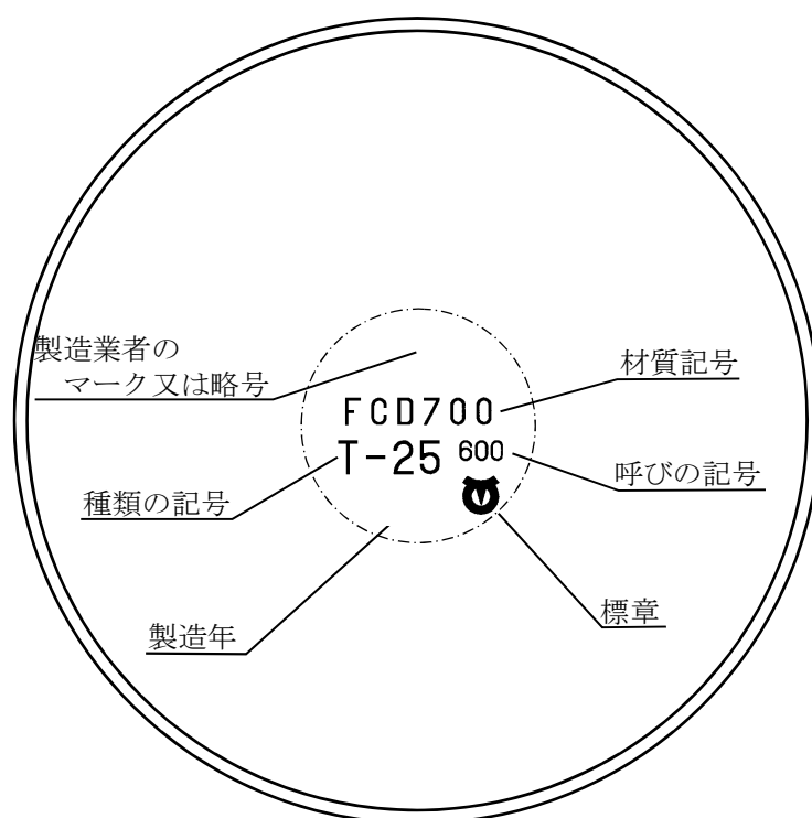
蓋裏面図
