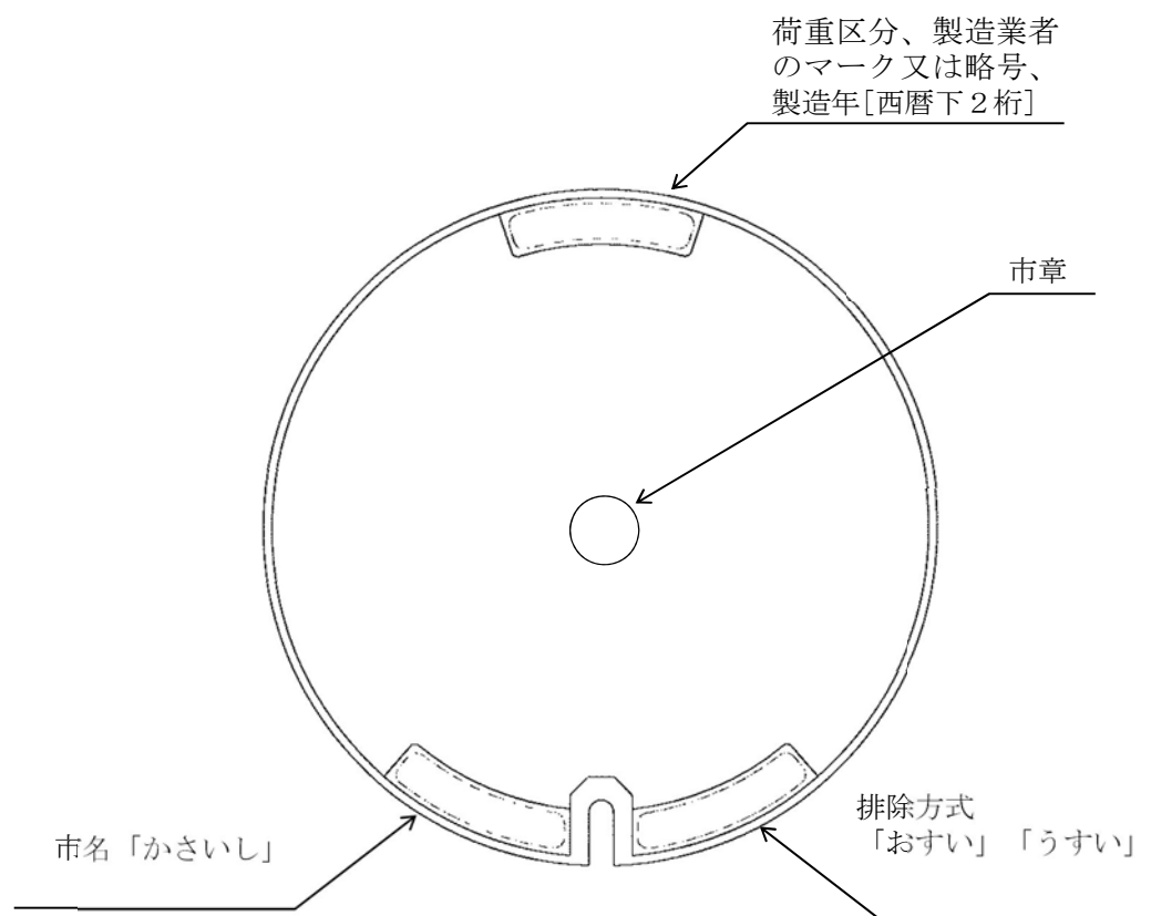
蓋表面図
