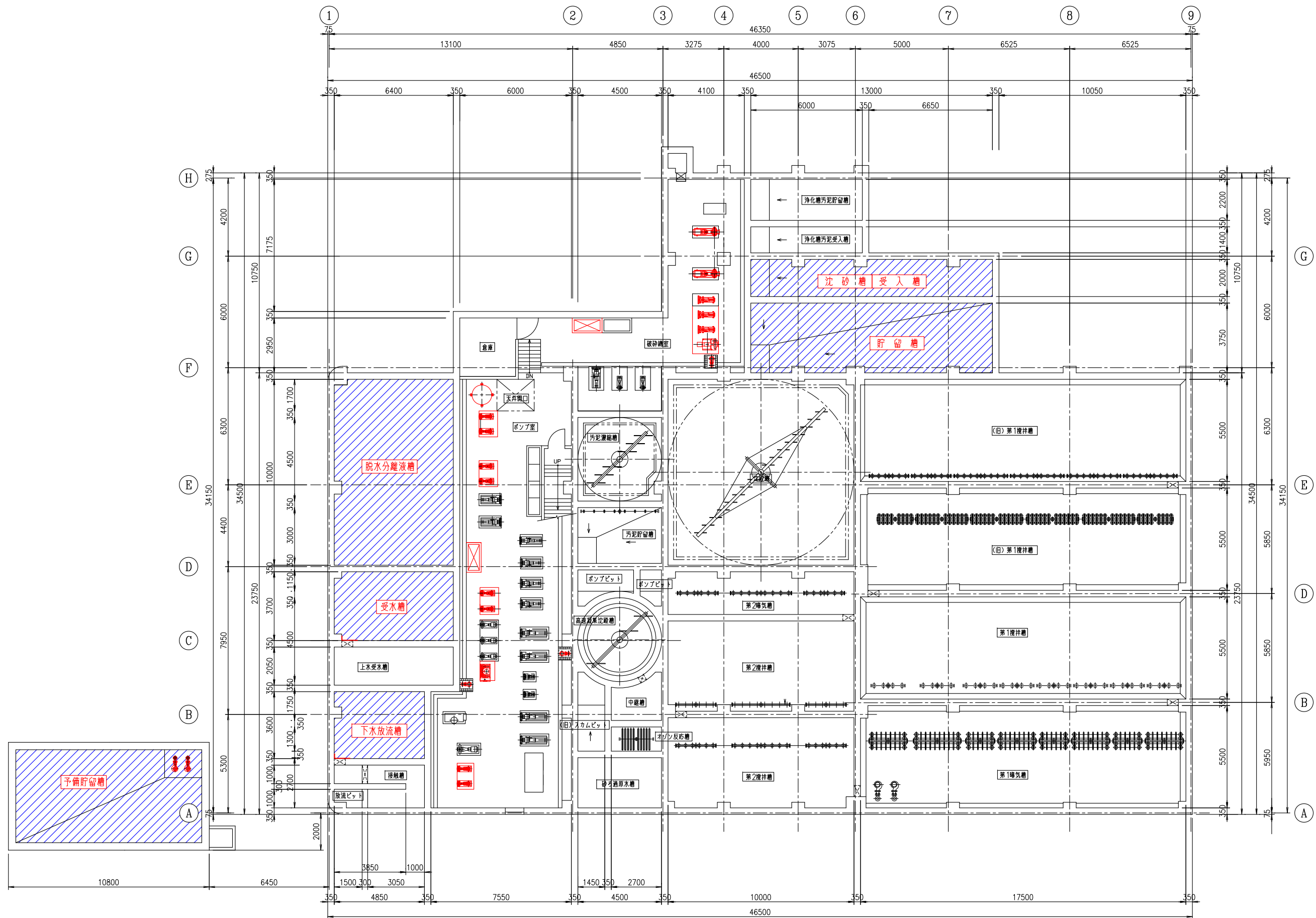
1階平面図
