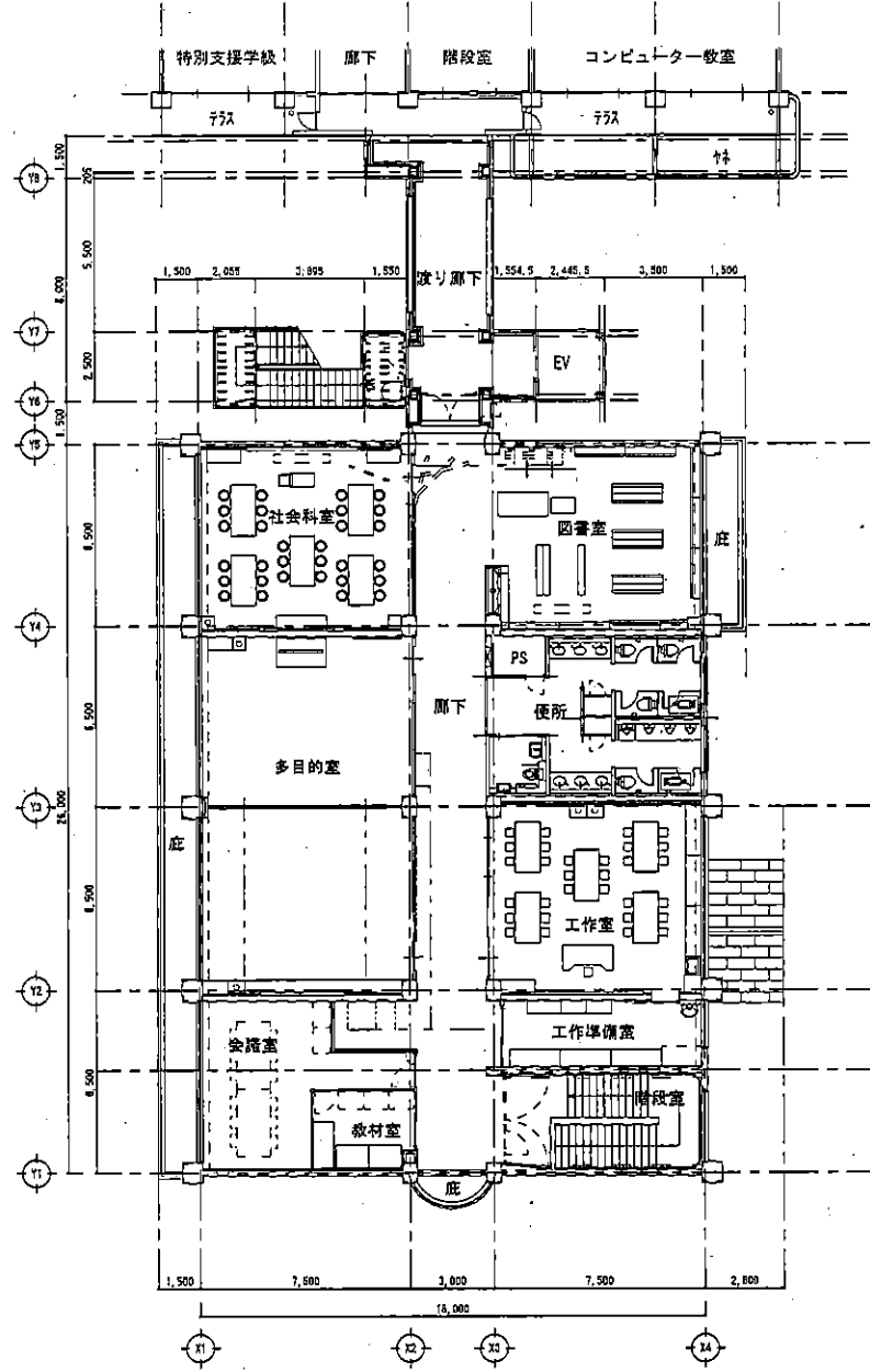
2 階平面図
