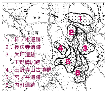
遺跡位置図
