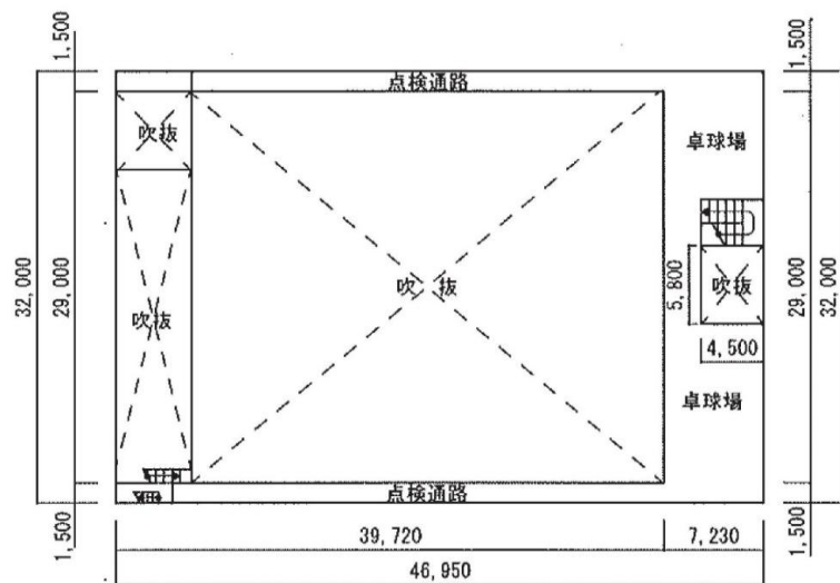
2F平面図
