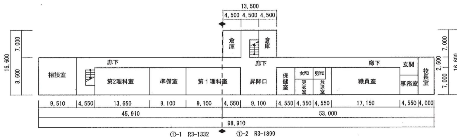
北棟 1F平面図
