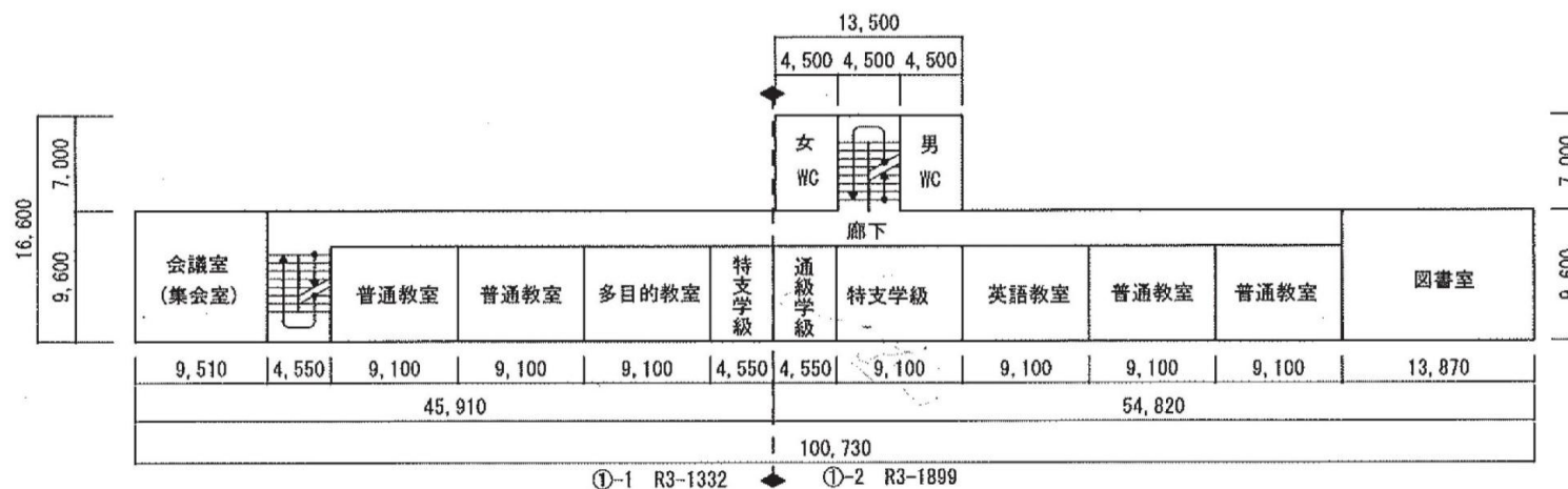
北棟 2F平面図
