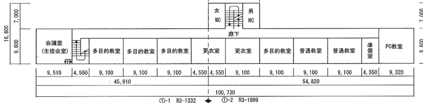
北棟 3F平面図
