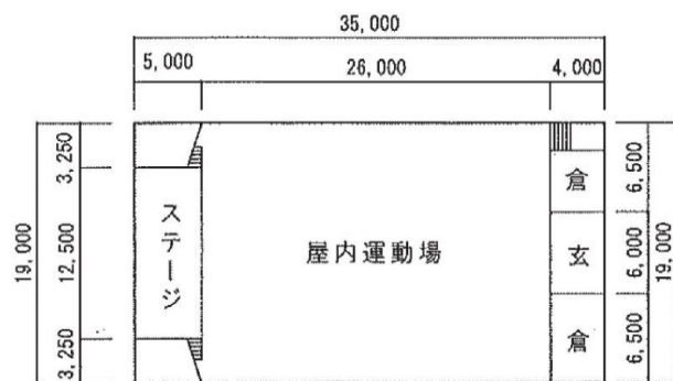
1階 平面図 ⑬ S2-825
