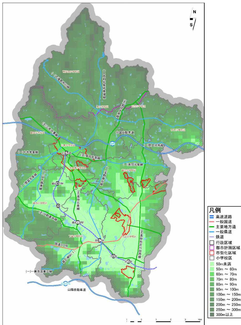
■図-* 標高5次（250m）メッシュで表示した加西市の地形 資料：国土数値情報
