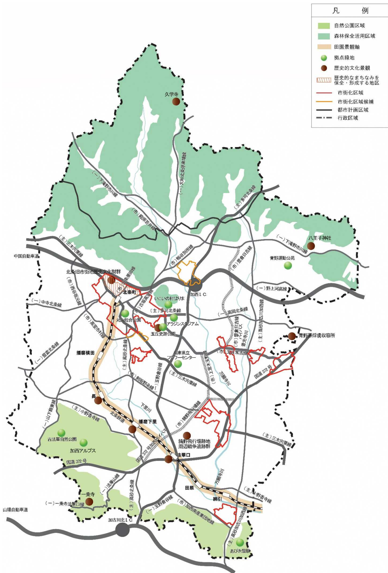
■図-77 自然環境保全・景観形成の方針図
